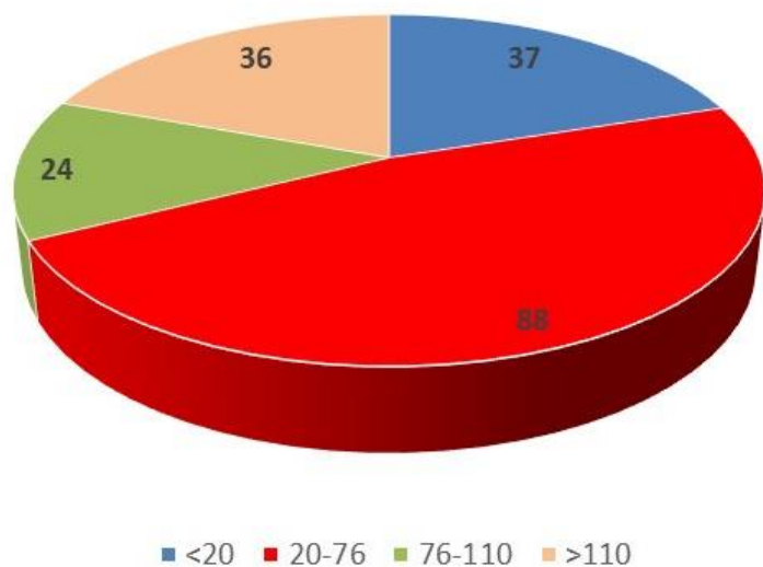
COORTE 2019-2020 III ANNO
