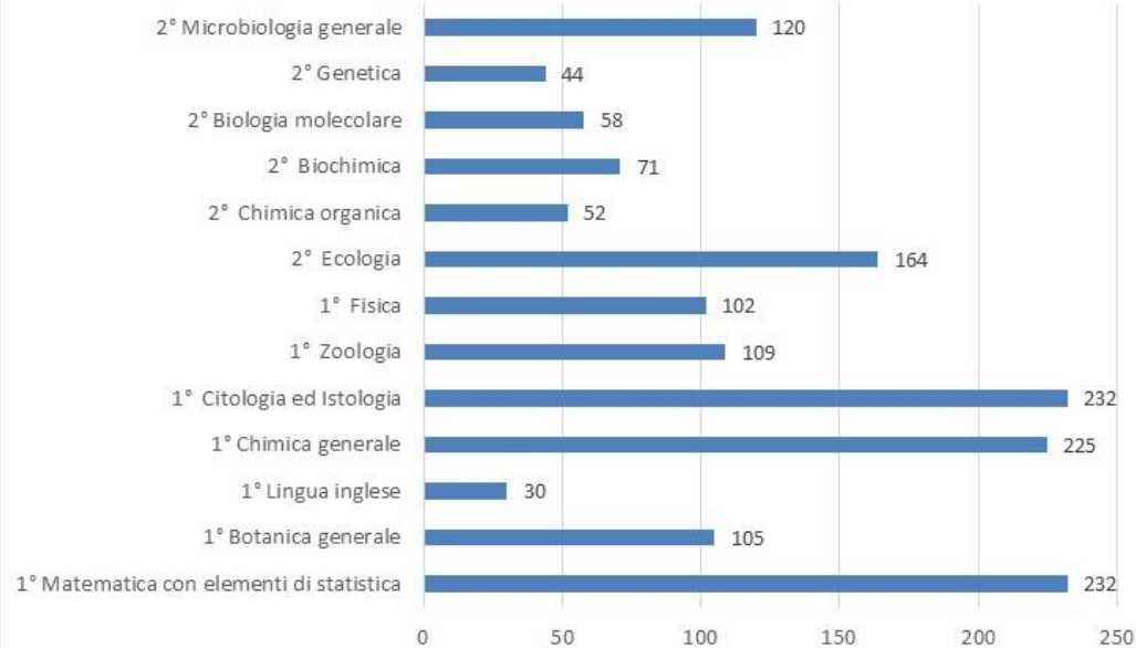
COORTE 2020-2021 II ANNO
