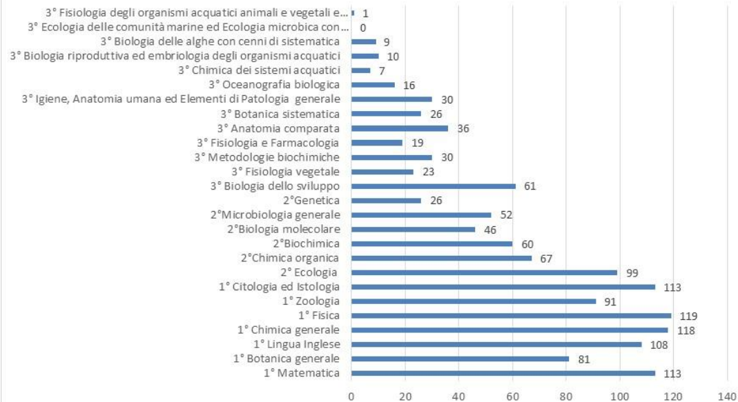
COORTE 2019-2020 III ANNO
